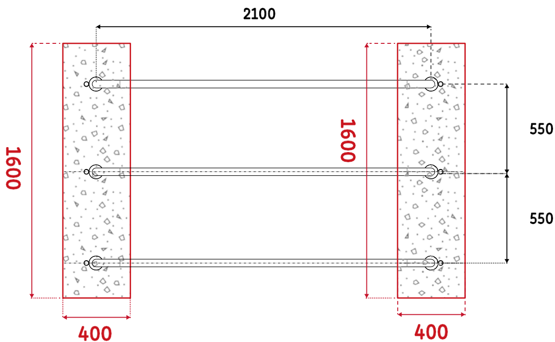
VISTA DALL'ALTO
