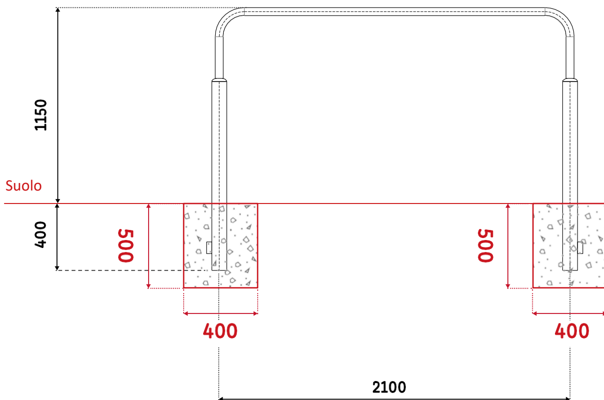
VISTA LATERALE
